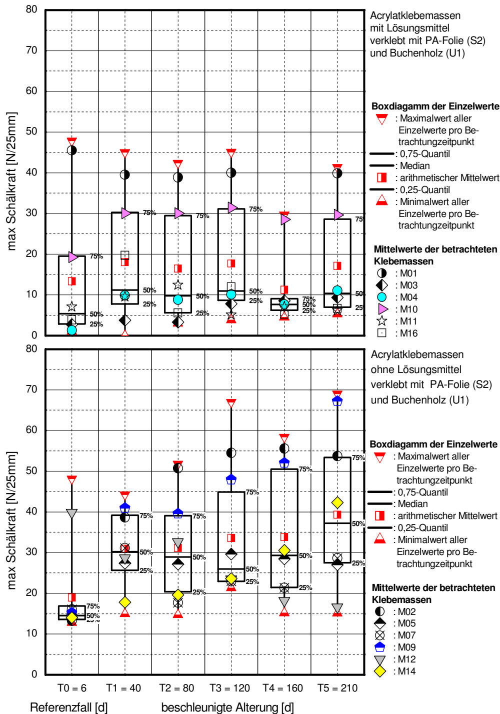
Bild 4: für jeden Konditionierungszeitpunkt ist ein Boxdiagramm dargestellt. Unterschieden werden Klebmassen mit und ohne Lösungsmittelanteil. Die Messwerte sind nach Dauer und Art der Konditionierung gegliedert T0 = Referenzfall, T1 bis T5 sind Konditionierungszeitpunkte der beschleunigten Alterung. Verklebt ist die Bahn S2 (PA - Folie) sowie der Untergrund U1 (Buchenholz).
